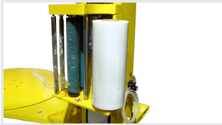
FA-Serie Integrierte Pre-Stretch Funktion Die Wickelfolie kann bis zu 300% gedehnt werden, um die Stabilität zu erhöhen und Folie zu sparen.
